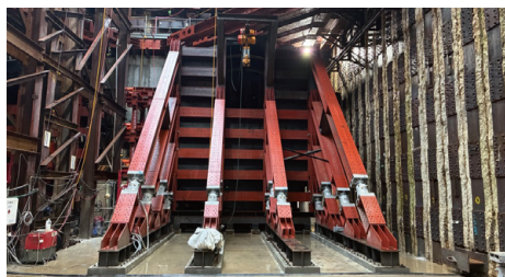
B 新井薬師前駅部 シールドマシン到達準備工事
