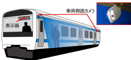
車載ホームモニタシステム（車両完結式）概要
