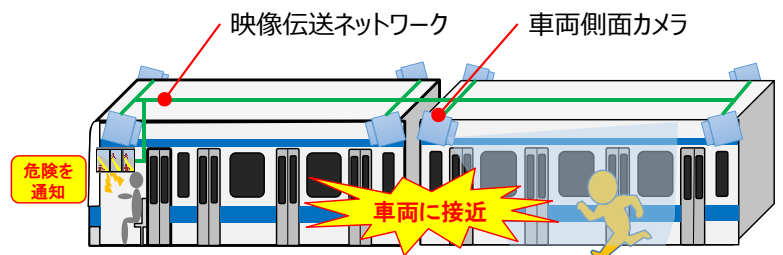
「お客さまの車両への接近を検知するシステム」 機能動作イメージ
